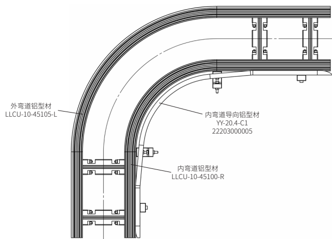
CU90 组装图
