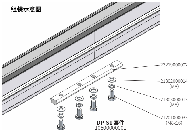
组装示意图
