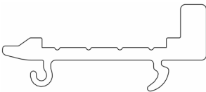
25 导向条 (有挡边)
