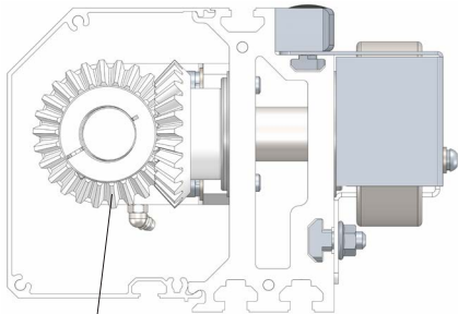
圆锥齿轮 26x2.5 10104000122
